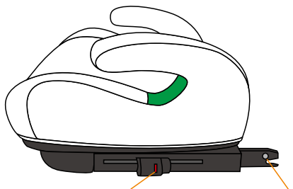
Botão de desbloqueio dos conectores ISOFIX
